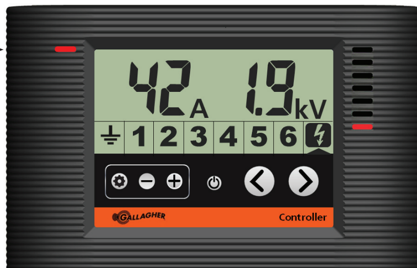
Elettificatore in allarme voltaggio d'uscita
